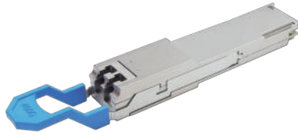
400G QSFP112-FR4
